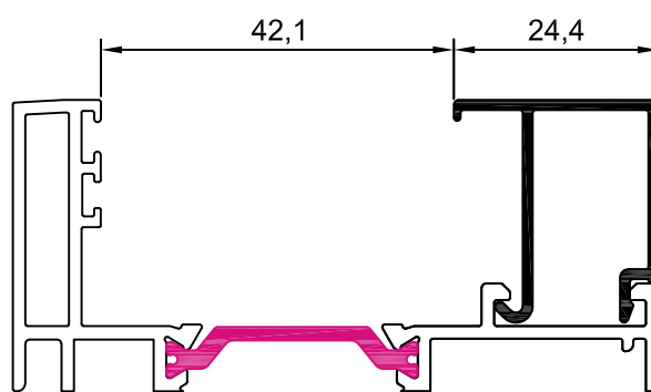
10006 junquillo 24,4 mm
