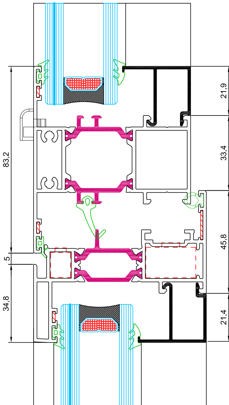
sección 6
