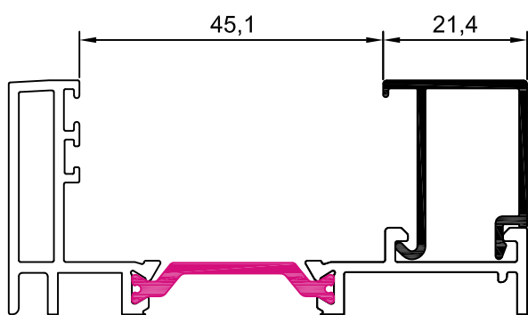
10005 junquillo 21,4 mm
