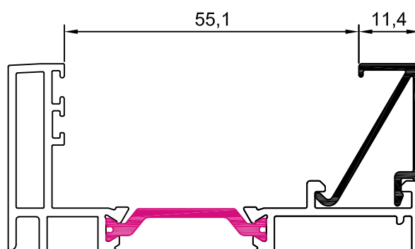
10002 junquillo 11,4 mm
